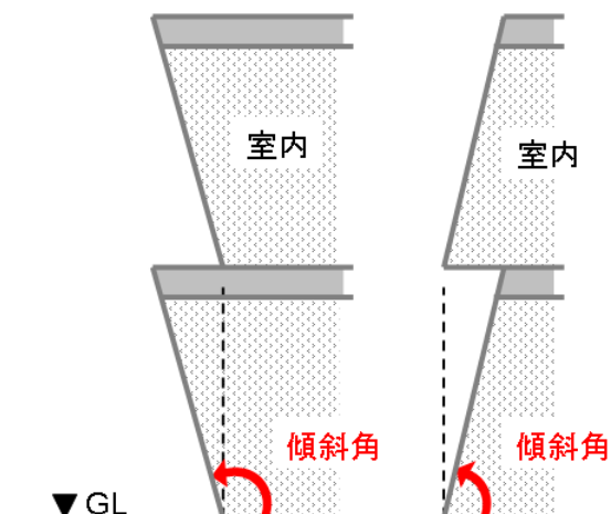
図 1.3.3.3 外壁の傾斜角
