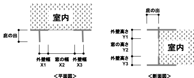
図 1.3.3.1-3 窓・庇の寸法入力
