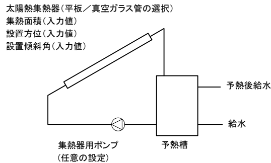
図 1.4.6.3-1 太陽熱給湯システム
