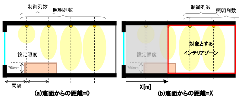
図 1.4.3.1-1 入力項目(断面概要図)
