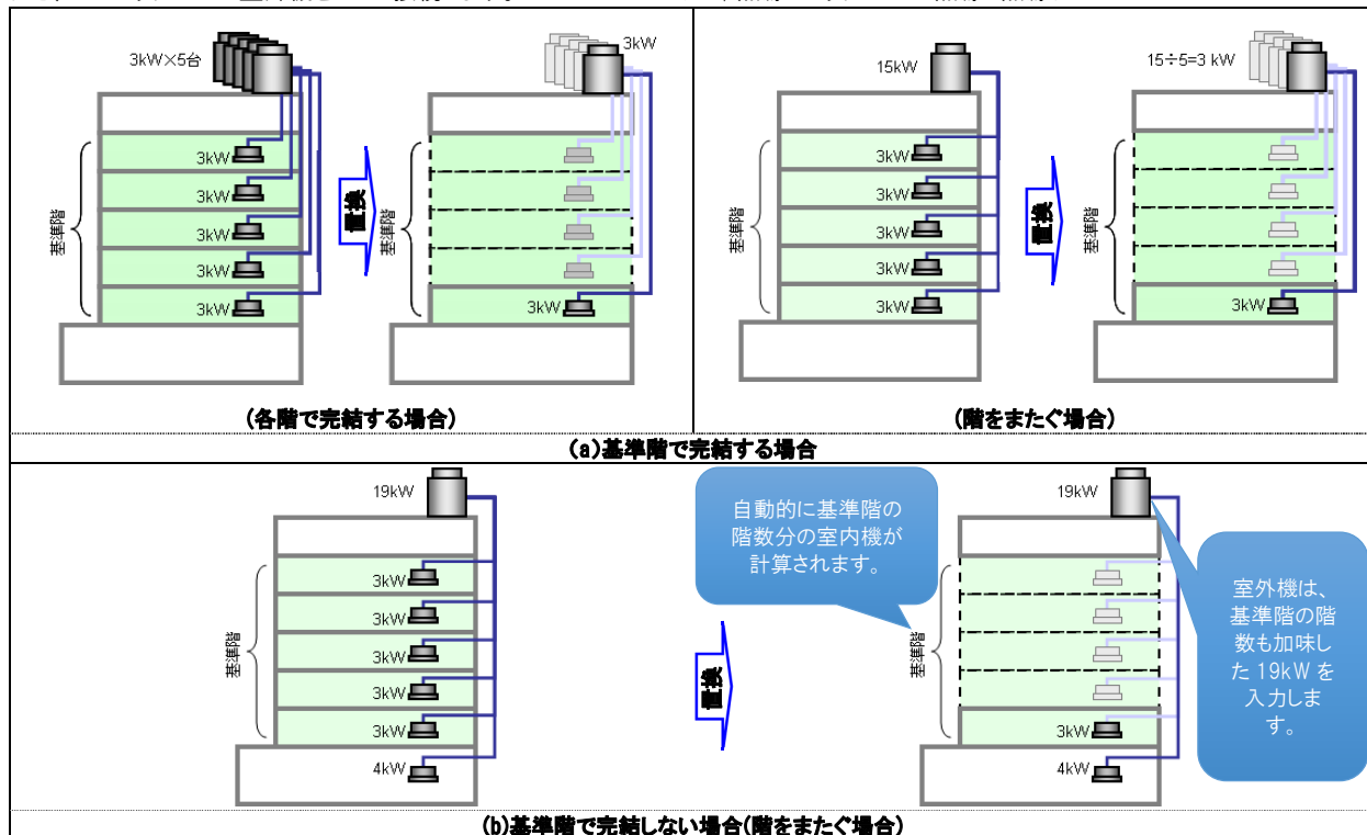
図 1.4.1.2-1 基準階の入力方法
