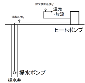
(熱交換器無し、井水槽なし)
