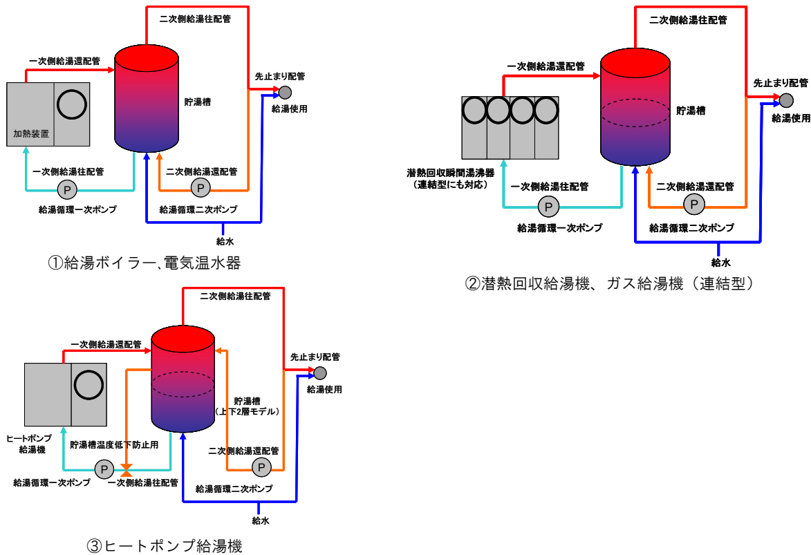
図 1.4.6.1-1 給湯システムのイメージ
