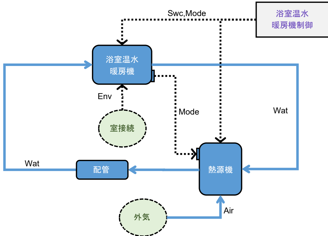
図1 温水床暖房
