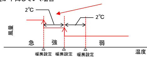
図2 ルームエアコンの室内機変風量制御ロジック
